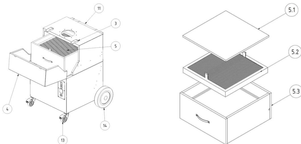
Fig. 14 : montage
