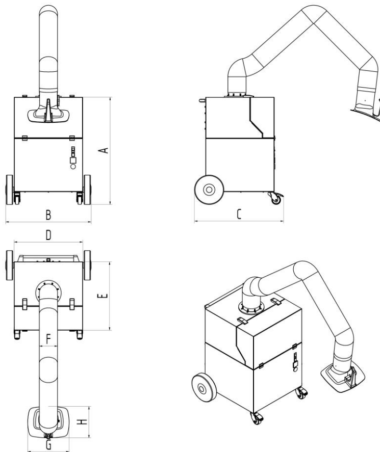
Afb. 24: Maatblad
