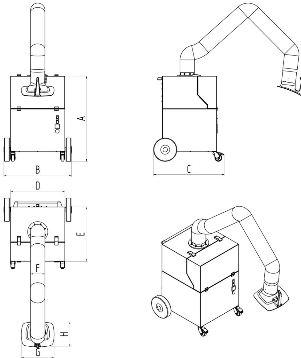
Abb. 6: Maßblatt
