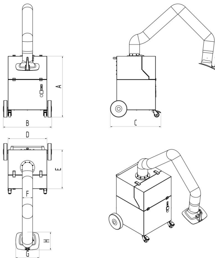
Rys. 54: Karta wymiarów
