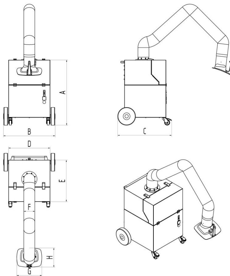
Fig. 18 : fiche dimensionnelle
