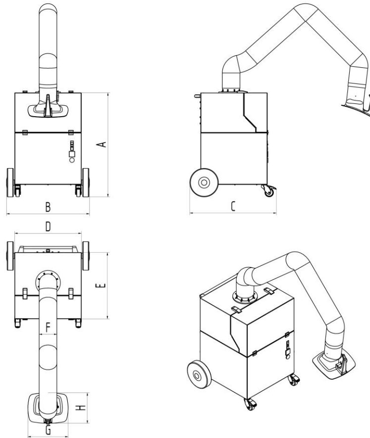
66. ábra: Méretlap
