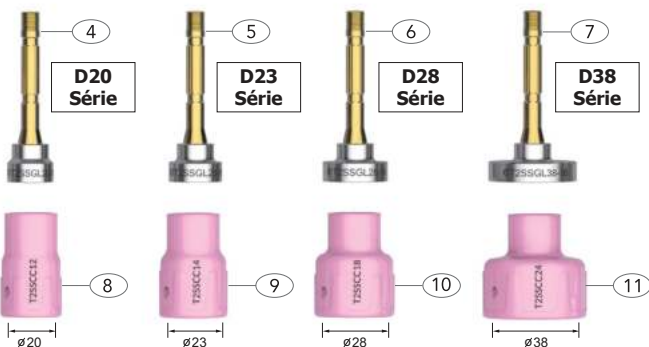
Hubice keramická
